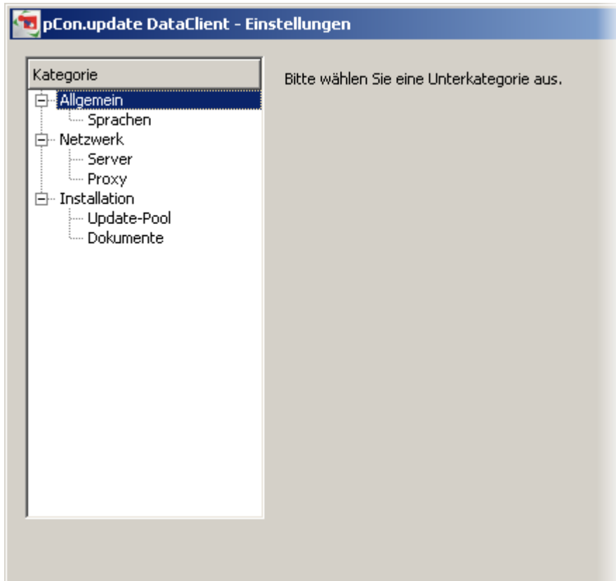
Einstellungsdialog
